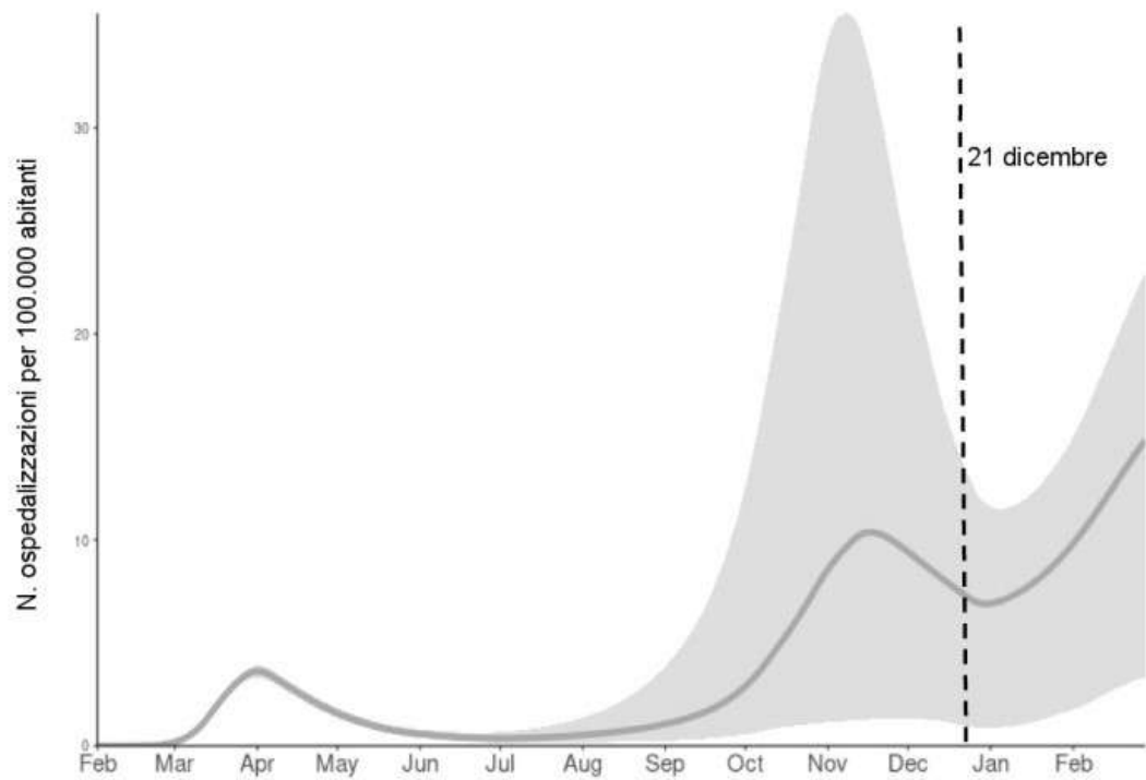
Revoca delle misure di restrizione il 21 dicembre 2020 (area grigia IC 95%)
