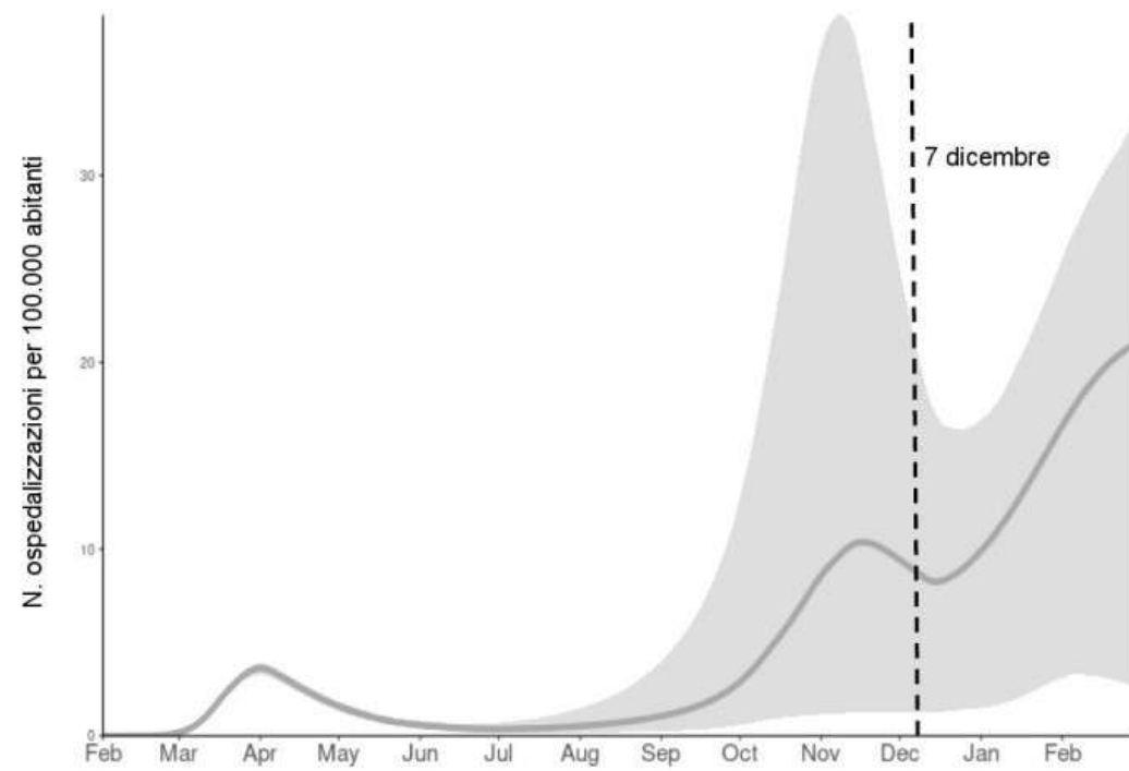
Revoca delle misure di restrizione il 7 dicembre 2020 (area grigia IC 95%)
